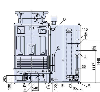
裏面図
