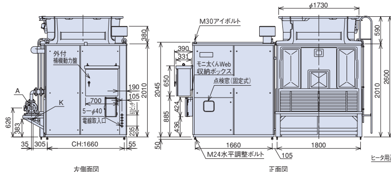
左側面図
