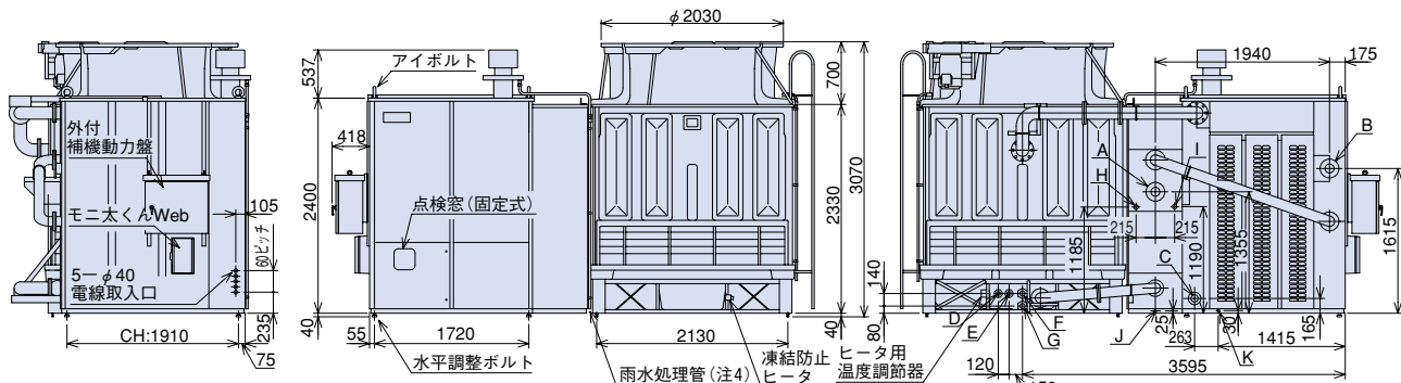
左側面図
