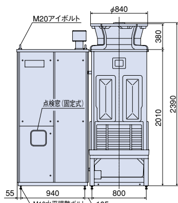
正面図
