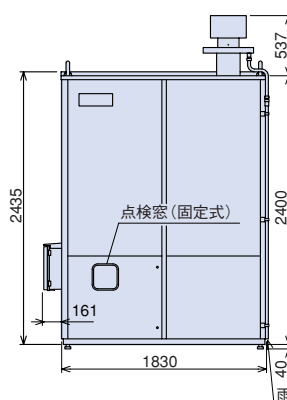
正面図
