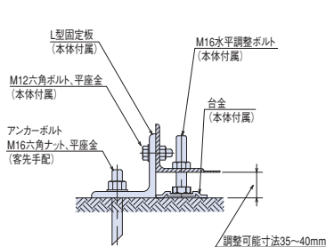
L型固定板取付図 (冷温水機)
