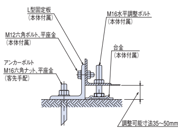
L型固定板取付図 (冷温水機)
