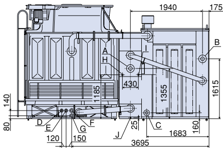
裏面図
