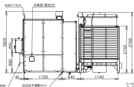
正面図
