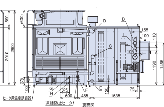
裏面図
