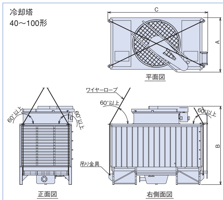
【搬入寸法】 (mm)
