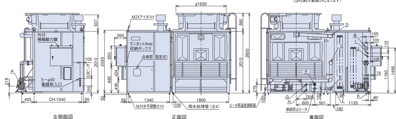
左側面図
