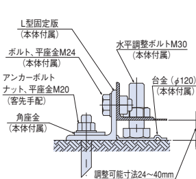
L型固定板取付図 (冷温水機)
