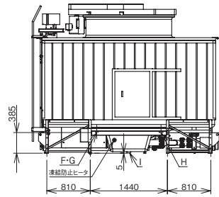
冷却塔右側面図
