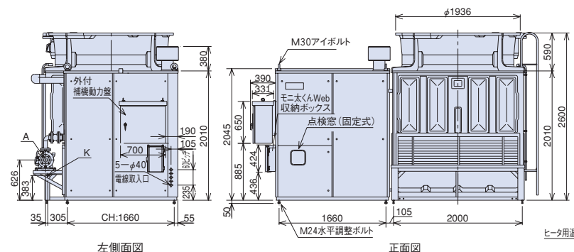
左側面図
