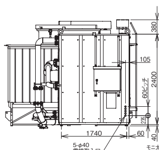
左側面図
