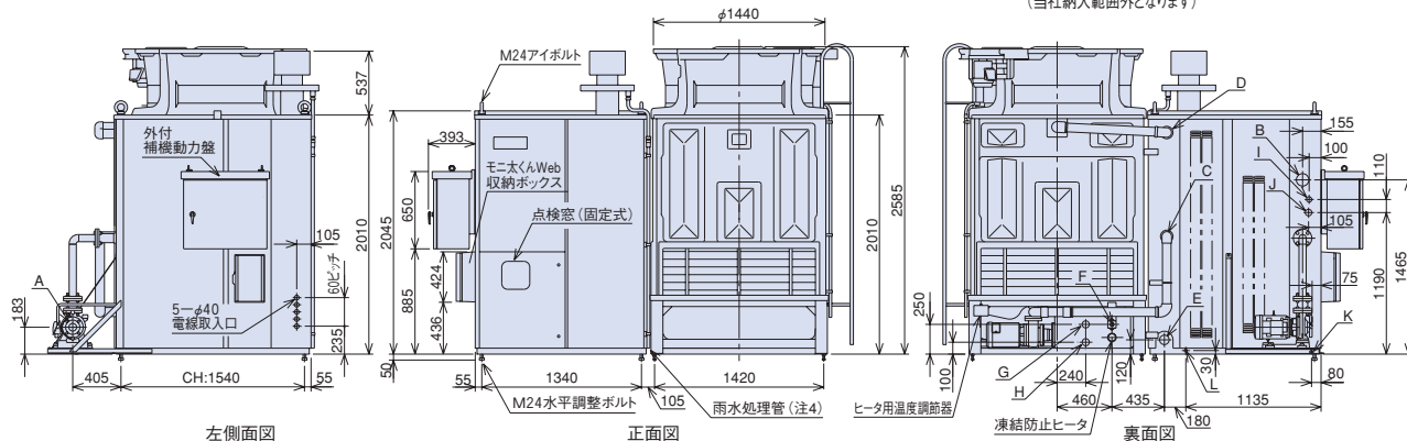
左側面図
