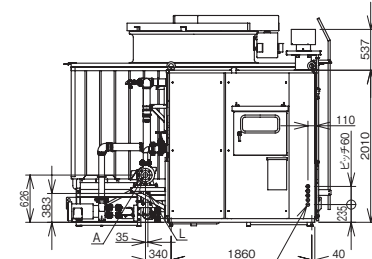
冷却塔右側面図
