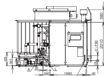
左側面図
