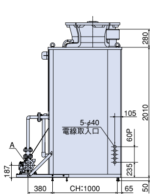
左側面図
