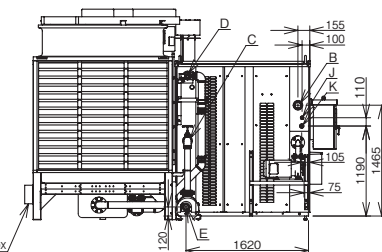
裏面図
