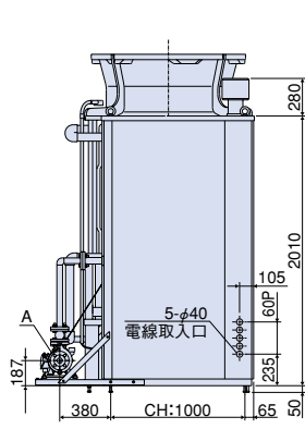
左側面図
