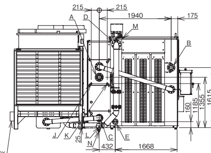
裏面図
