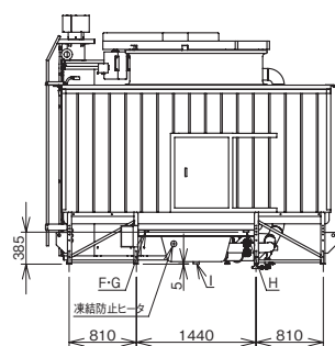
冷却塔右側面図
