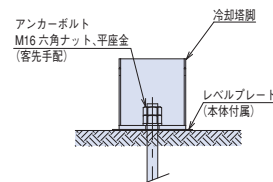
基礎固定参考図 (冷却塔側)
