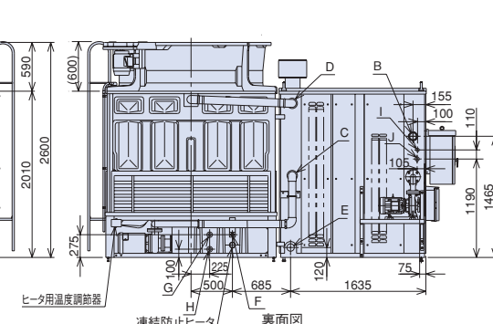
裏面図
