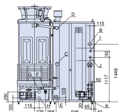
裏面図
