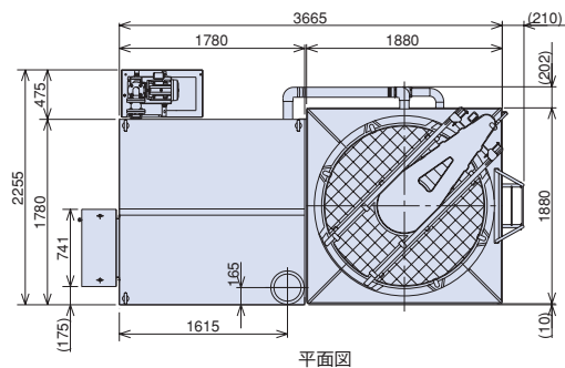
平面图
