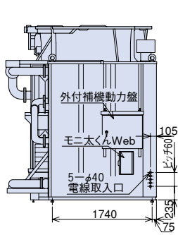
左側面図
