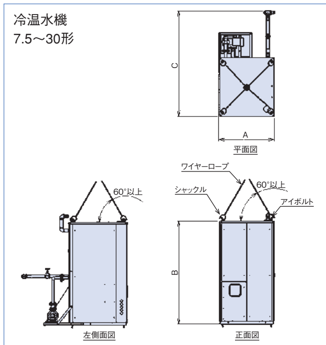
【搬入寸法】 (mm)
