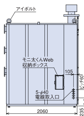
左側面図
