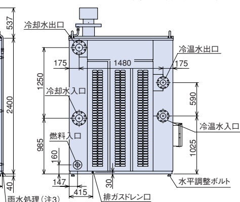
裏面図
