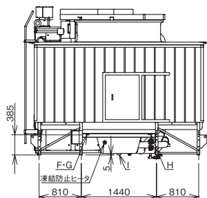
冷却塔右側面図
