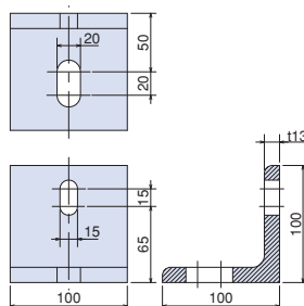
L型固定板 (冷温水機)
