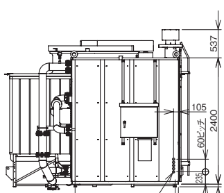
冷却塔右側面図
