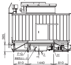
冷却塔右側面図
